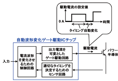
自動波形変化ゲート駆動 IC チップ
