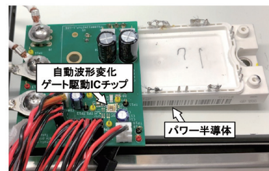
自動波形変化ゲート駆動 IC で パワー半導体を駆動する測定系
