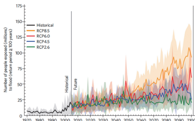
大規模な洪水に対するリスク人口の将来予測
