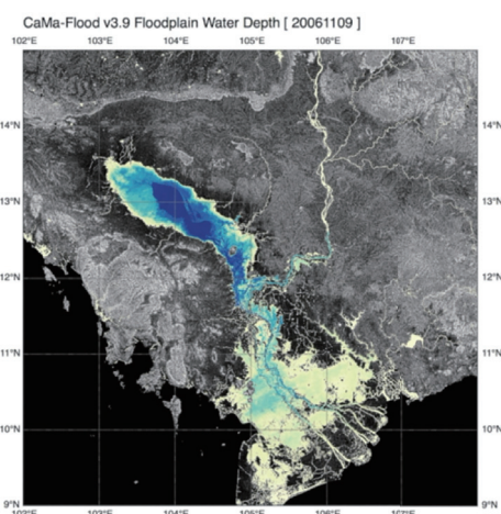
グローバルな洪水リスクマップのためのモデル開発
