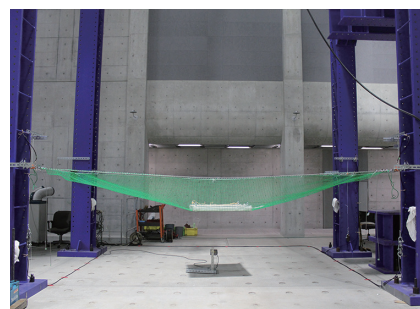
落下防止ネットへの天井板の落下実験
