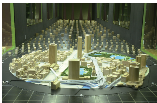
環境無音境界層風洞
