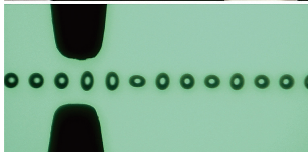
液体表界面の状態変化を空中飛翔液滴の振動観察によって追跡！マイクロ秒の時間分解能を有する「表界面現象モニター装置」
