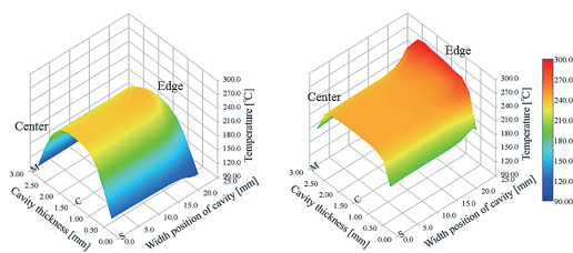
(a) Injection rate 10cm³/s (b) Injection rate 100cm³/s キャビティ流動樹脂内部の3次元温度分布計測（材料：PP）
