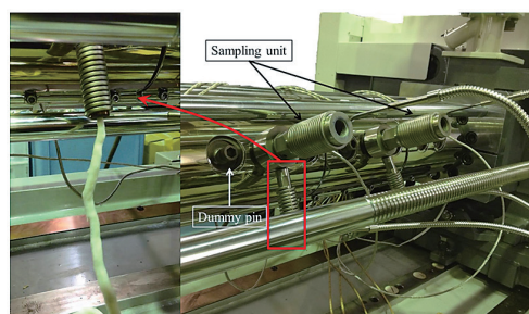
可塑化樹脂のインプロセス多点サンプリング装置
