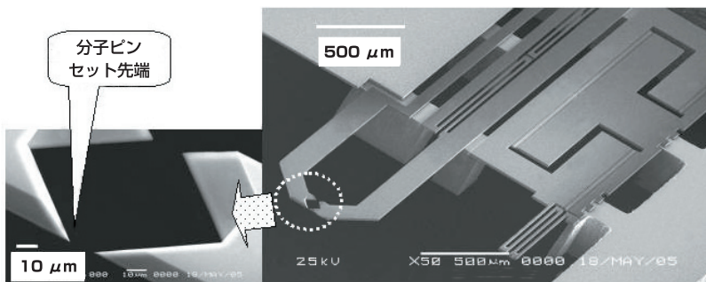
ミクロのピンセット。厚みは20 \mu\text{m} 。
