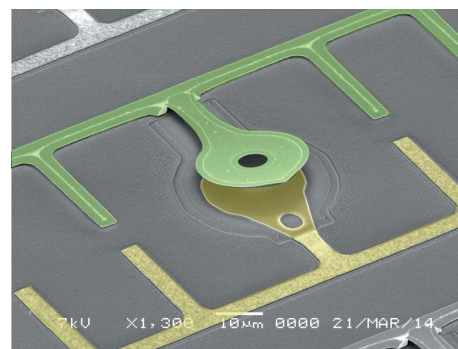
THz波の空間変調用 可動LC共振器
