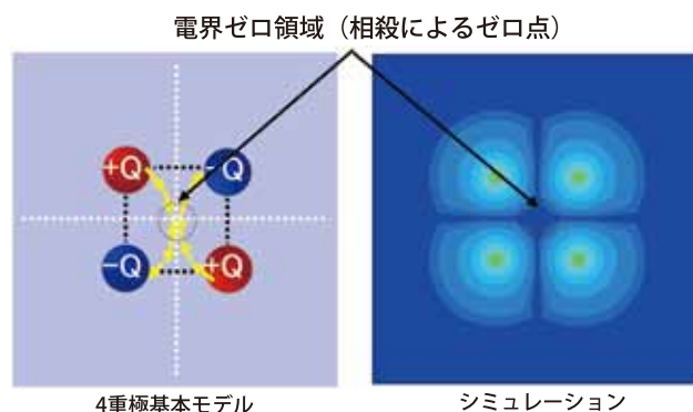
多重極構造による基準電位生成
