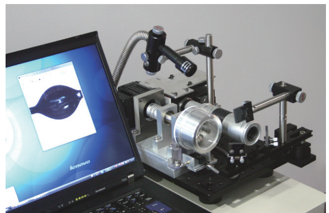
「あらゆる液体の計測を可能にする レボルピング・ドロップ表面張力計」
