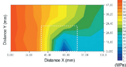
(2) 圧力分布
