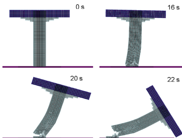
応用要素法 (AEM) によるRC橋脚の崩壊挙動シミュレーション
