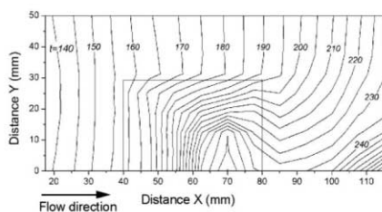
(1) 充填パターン (t: 充填時間 (ms))
