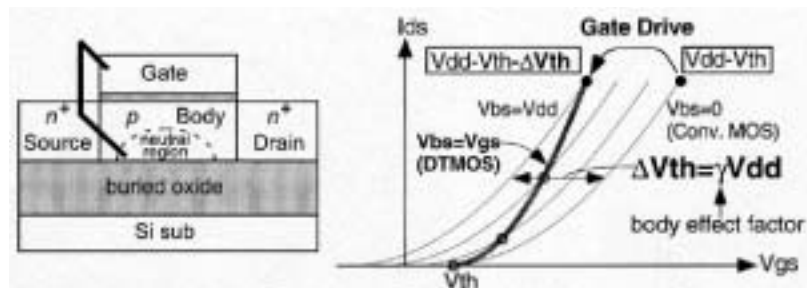
Dynamic Threshold MOSFET (DTMOS)
