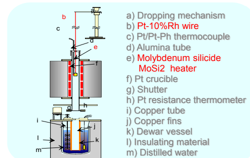
図4. 1600 まで使用可能な高温落下型熱量計
