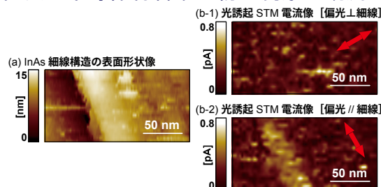
光照射STMIによるInAs細線上での光誘起電流信号の獲得
