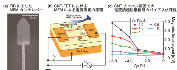
MFM電流誘起磁場計測系によるカーボンナノチューブFETチャネルの評価
