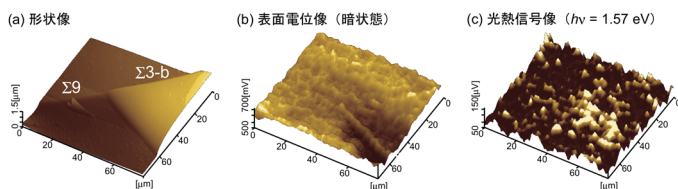
多結晶シリコン太陽電池における形状／表面電位／光熱信号分布
