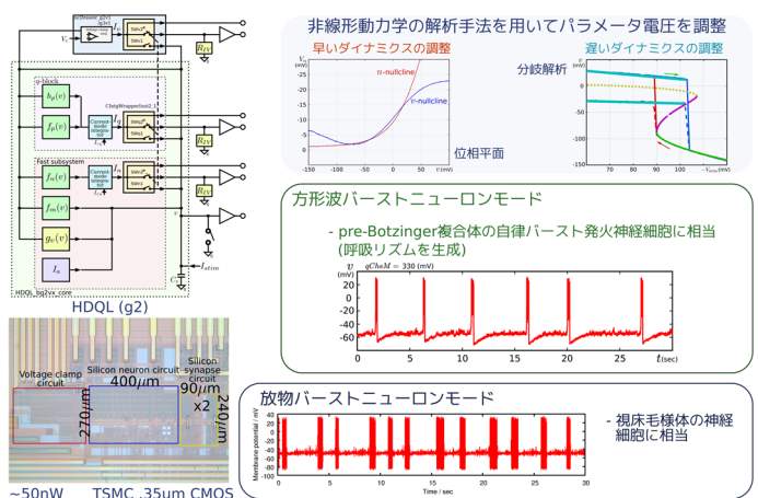
図2. プログラマブルシリコンニューロン回路
