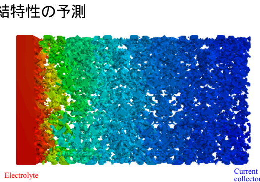
図2 格子ボルツマン法により計算された燃料極内酸化物イオン電気化学ポテンシャル分布
