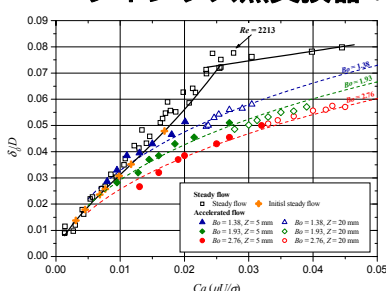
図4 加速流れ中の液膜厚さ
