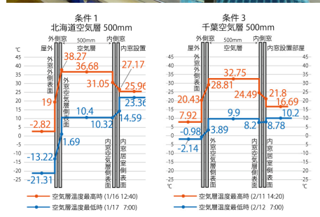
太陽光輻射による内窓集熱実験
