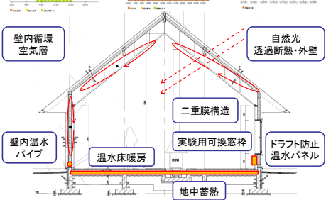
寒冷地実験住宅 モニタリング
