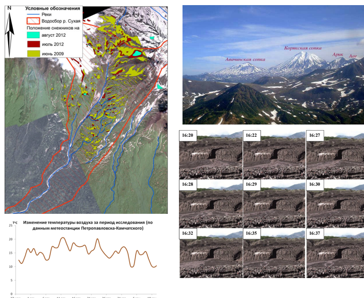
図2. カムチャツカ火山群における環境変動の観測および予測
