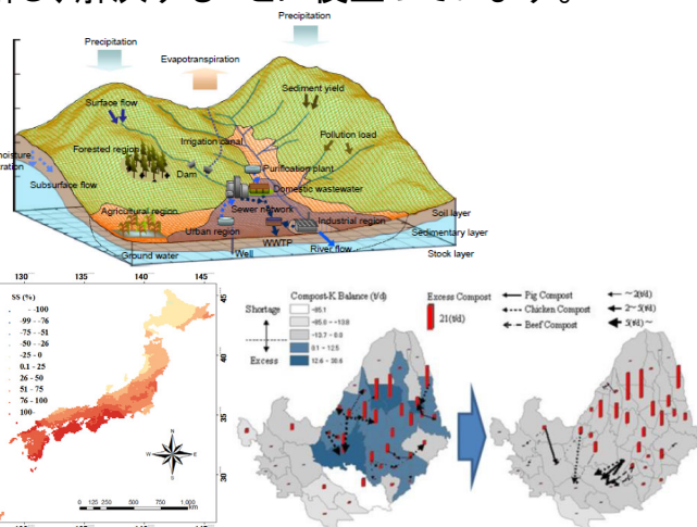
図1. 本研究により構築された水利用システムによる環境変動の予測
