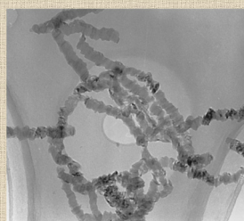
プレートレットカーボンナノファイバー
