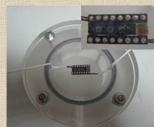
プレートレットカーボンナノファイバーを利用したアンモニアガスセンサー
