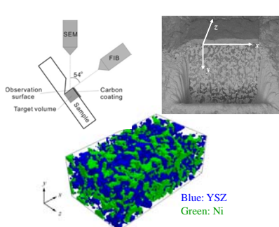
図1 Dual Beam Focused Ion Beam-Scanning Electron Microscopeによる電極3次元構造の計測
