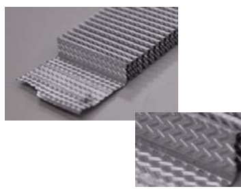
図5 層流域での熱物質促進を図った斜交波状フィン
