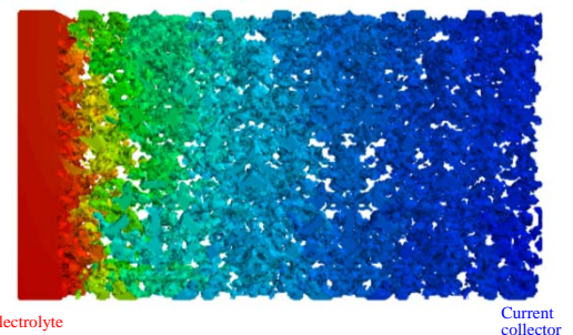
図3 格子ボルツマン法により計算された燃料極内酸化物イオン電気化学ポテンシャル分布
