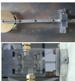
図4 単管振動流蒸気サイクル試作機
