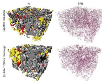
図2 通電による燃料極ニッケル構造と三相界面の変化
