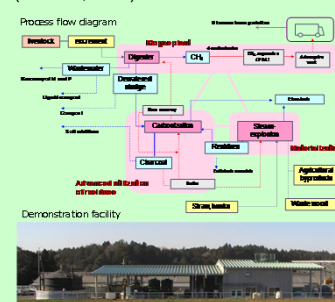
Demonstration of Local Biogas Utilization (Katori-shi, Chiba)
