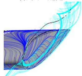
図2 翼端漏れ渦の可視化
