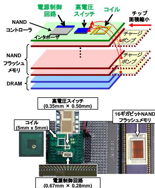
三次元Solid-State Drive向け新電源システム
