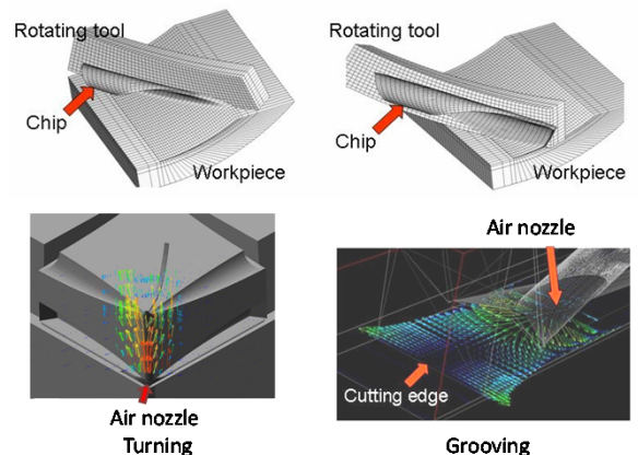
エンドミル切削(上図)とMQL切削(下図)
