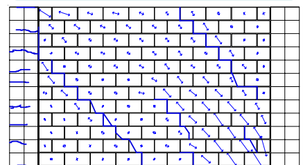
ブロック造壁の主圧縮歪度分布
