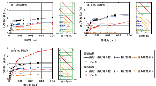
ひび割れ長さ推定結果と実験結果の比較
