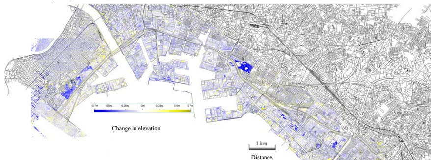
図2(左). 液状化による浦安の地盤沈下の計測(朝日航洋との共同調査)：震災前(2006年12月～2007年1月)、震災後(2011年4月20日(浦安)、9月6日、12月28日(市川～千葉))の地形計測データを用いて差分計算することで、東京湾岸地域の液状化による地表面沈下を抽出した。杭支持の建物屋上や首都高湾岸線の橋脚標高が変わらないものとした。(日本学術振興会科学研究補助金(23246087)、生産技術奨励会支援経費による)
