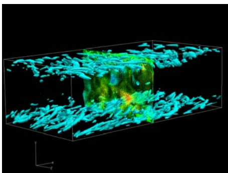
図1 チャンネル乱流の壁近くの渦
