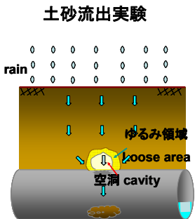
埋設管破損による土砂流出と空洞形成
