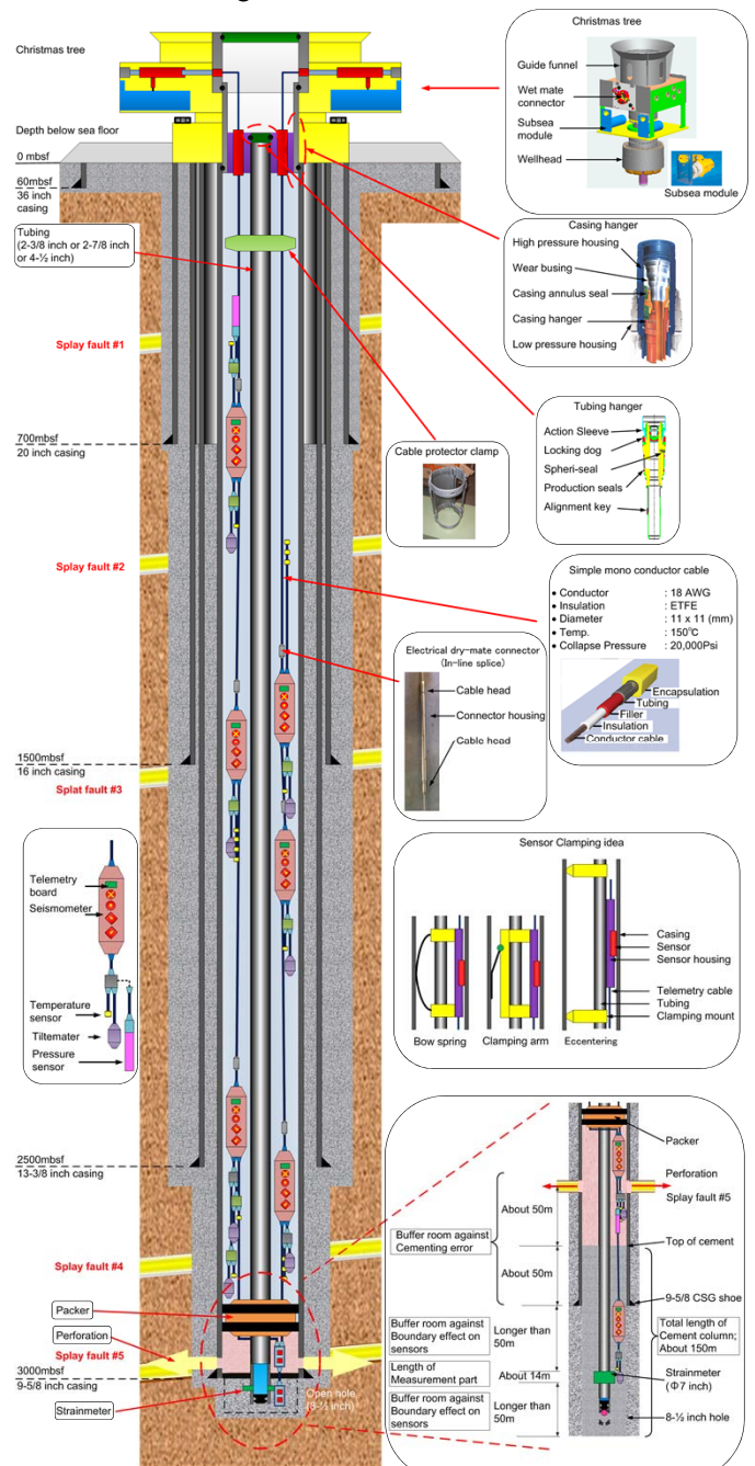
図1 3.5kmライザ孔用長期孔内観測システムの概念
