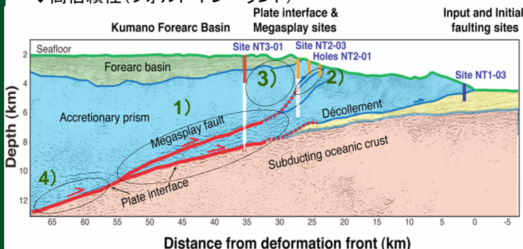
図2 南海トラフ地震発生帯における長期孔内観測の科学目的
