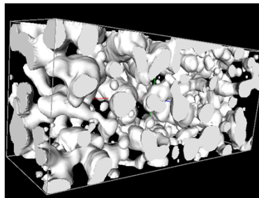
図2 レベルセット法による燃料極ニッケル表面の等値面表示
