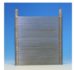
図7 SUS製フィンレス熱交換器
