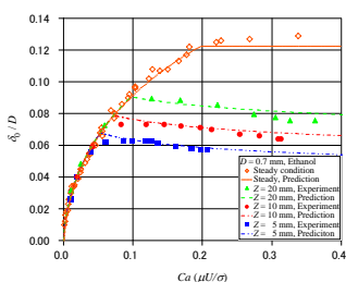
図4 細径管内二相流液膜厚さの測定
