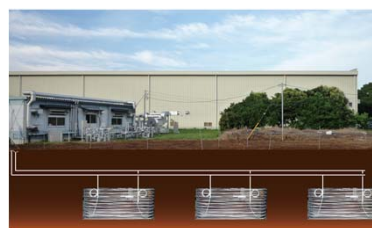
省エネ型都市交通システム「エコライド」試験設備
