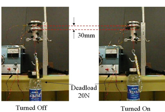
強磁性形状記憶合金アクチュエータの磁場・超弾性応答
