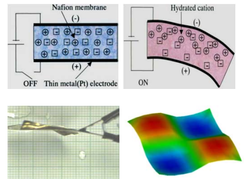
導電性高分子アクチュエータの電気化学・力学応答
