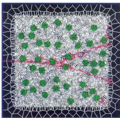
2相材料の損傷・破壊 (アルミナ+ジルコニア粒子)
