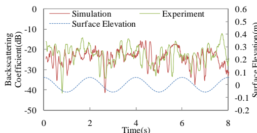
マイクロ波後方散乱係数
