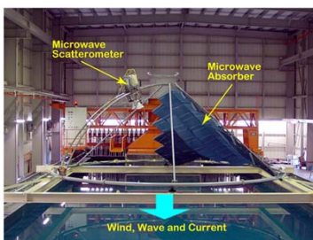
マイクロ波後方散乱計測システム
