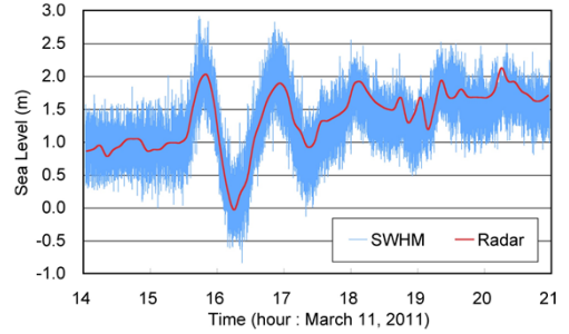
レーダが計測した2011年3月11日の津波
