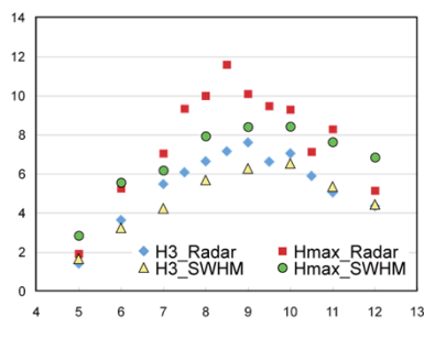
パルスドップラーレーダが計測した2009年台風18号通過時の平塚沖波浪
