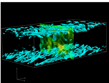
図1 チャンネル乱流の壁近くの渦
