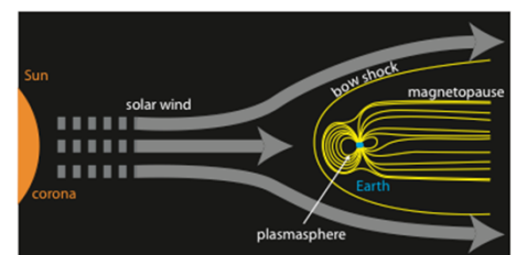
図3 太陽風と地球磁場
