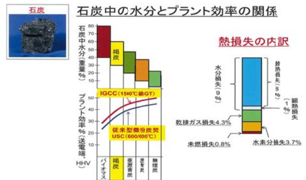
石炭の種類と熱効率
