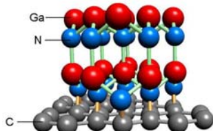
グラファイトシートと窒化ガリウム薄膜のヘテロ界面における原子配列
