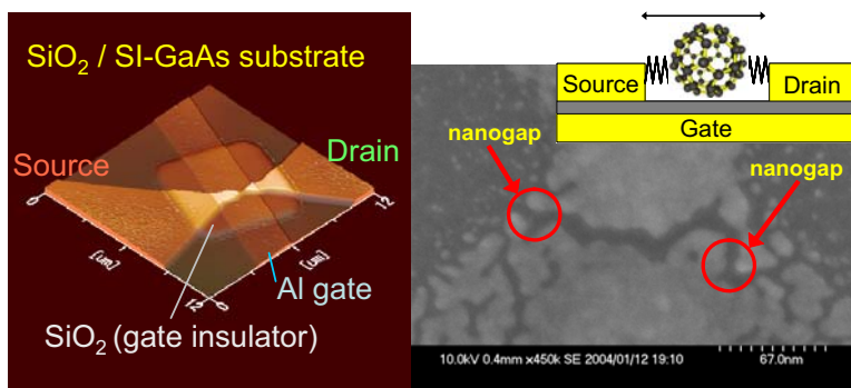
原子レベルのナノギャップを有する電極の作製と単一分子をチャンネルとするトランジスタの作製
