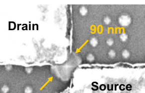
単一の自己組織化InAs量子ドットをチャンネルとする単一電子トランジスタの物理と応用
