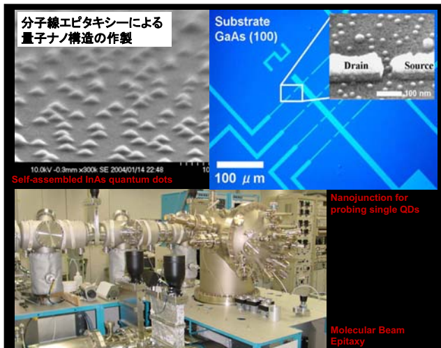
単一の自己組織化InAs量子ドットをチャンネルとする単一電子トランジスタの物理と応用
