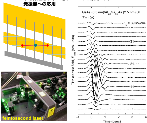
半導体超格子中の電子のプロッホ振動とテラヘルツ発振器への応用
