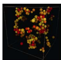
ガラス形成液体に見られる中距離結晶秩序
