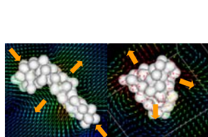
高分子鎖の凝縮転移時の流れ場の様子
