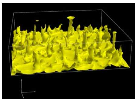
回転系の熱対流乱流の上昇プルーム
