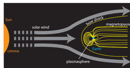
太陽風と地球磁場
