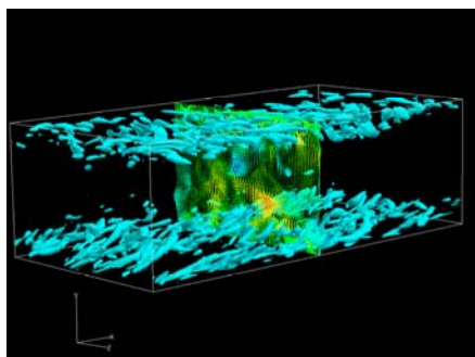
チャンネル乱流の渦と断面の速度
