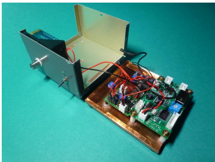
制御回路
