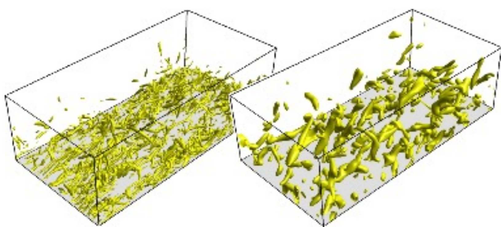
図1 チャンネル乱流の壁近くの渦構造
