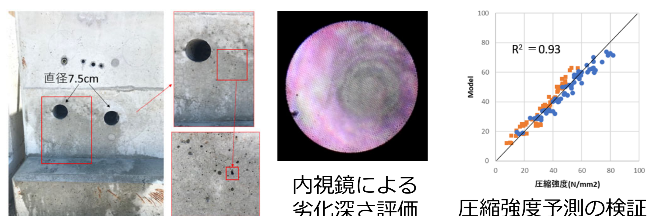
圧縮強度予測の検証
