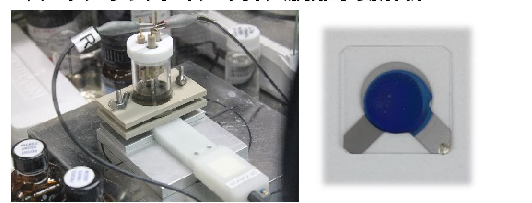
電気化学水晶振動子マイクロバランス法を用いたマグネシウムイオンの挿入脱離挙動解析
