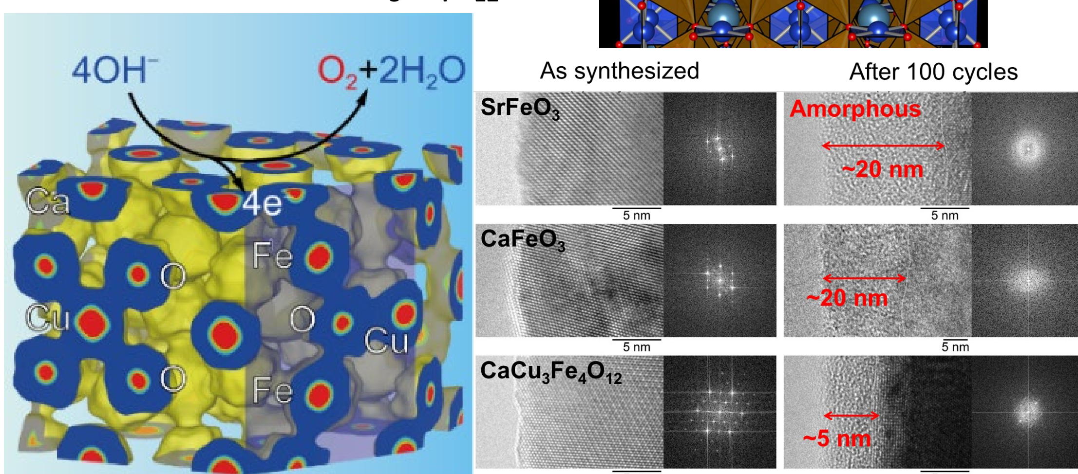
酸素発生反応に対して高い活性を有する酸化物触媒CaCu 3 Fe 4 O 12
