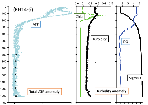
マリアナトラフ Seamount-Xにおける鉛直ATP計測の結果。ATP定量分析装置をCTDに搭載して計測
