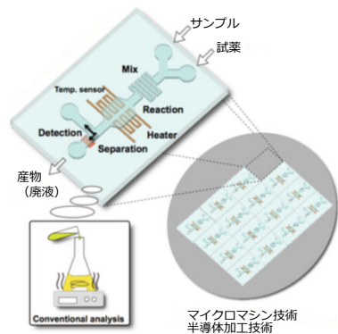
マイクロ流体システムの概念図
