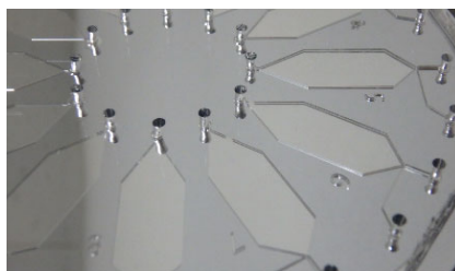
微生物DNA精製用マイクロ流体デバイス (金研究室と共同)
