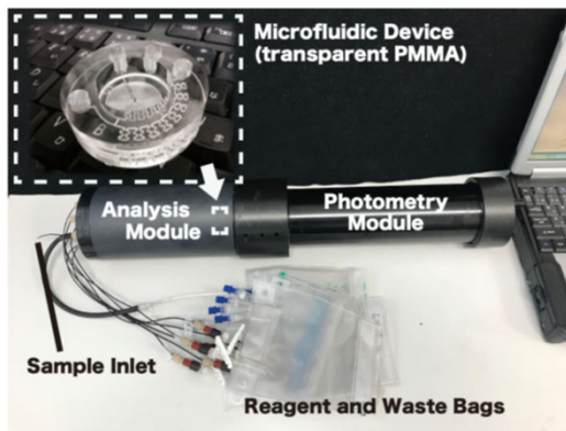
現場型 ATP 定量分析装置の外観 Fukuba et al., Micromachines 2018
