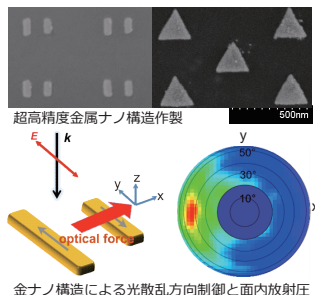
金ナノ構造による光散乱方向制御と面内放射圧
