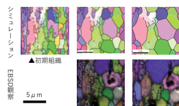
▲Al1050合金の再結晶挙動 実際の組織変化とフェーズフィールドシミュレーションを同化
