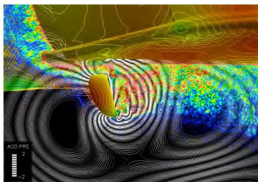
ドアミラーまわりの流れと音
