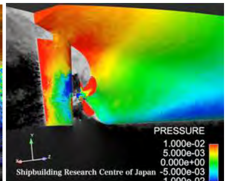
船体まわりの流れ
