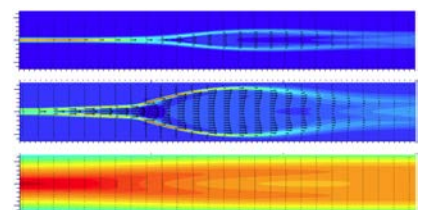
図3 磁気リコネクションのジェット
